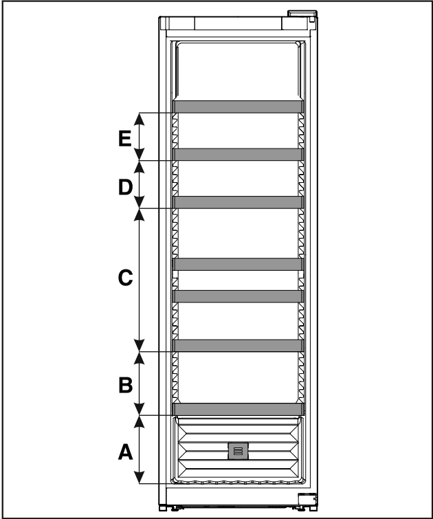
Fig. 59 Afstanden oplegroosters
