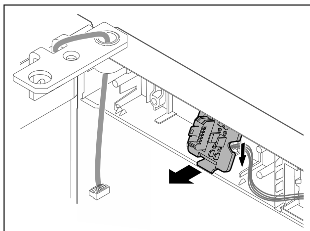
Fig. 9 De inbouwpositie van de stekkerhouder kan 180° gedraaid zijn.*
