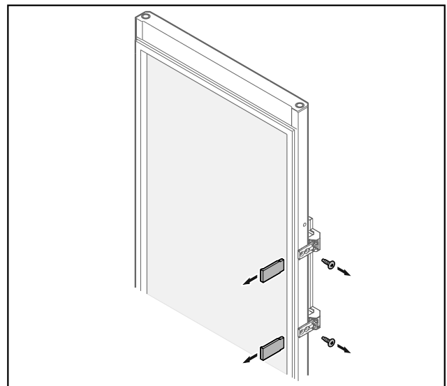
Fig. 17 Glasdeur
